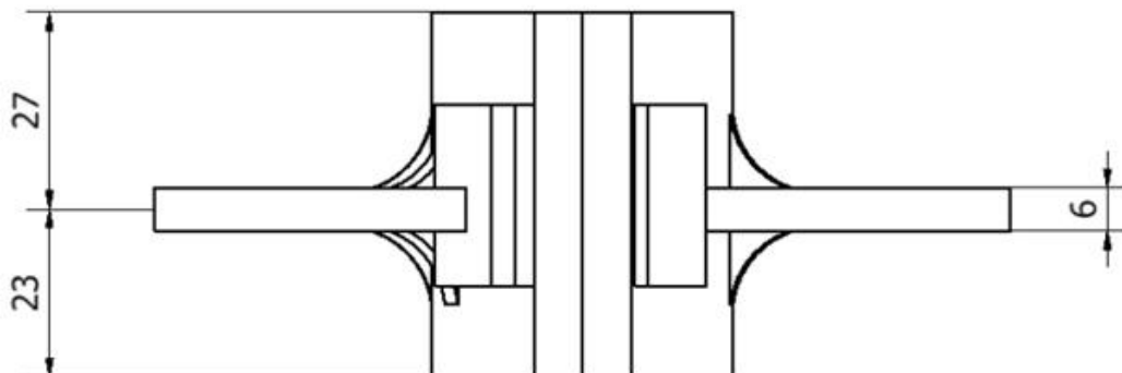
DETTAGLIO GIUNTO
